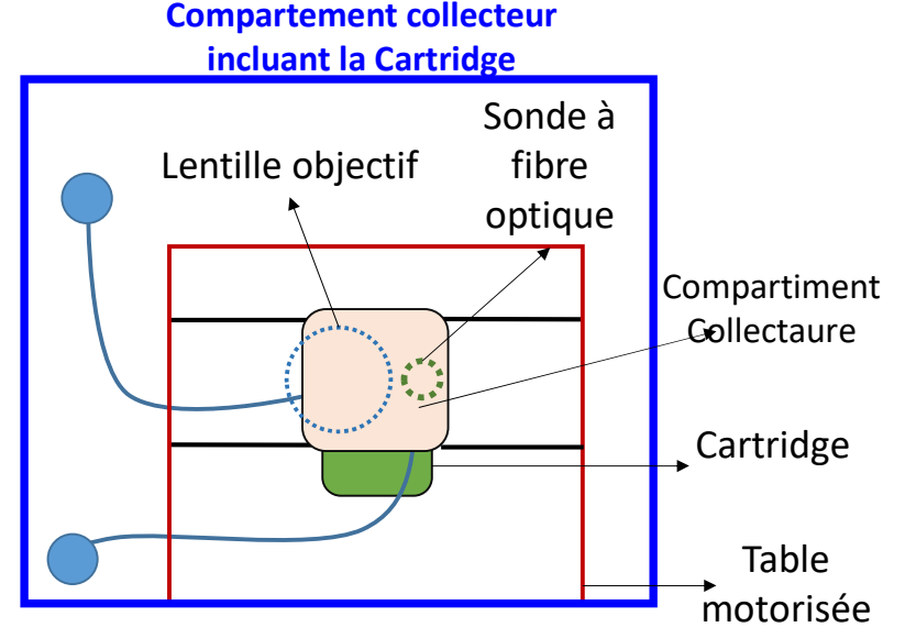
POSITION FERMÉE (pour UTILISATION CARTRIDGE)
